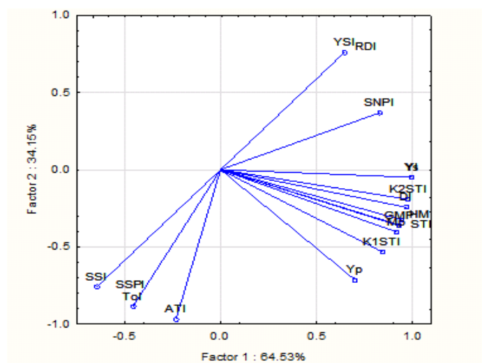
شکل ۱- نمایش شاخص های مقاومت به خشکی بر اساس دو مؤلفه اصلی در شرایط بدون تنش و تنش
